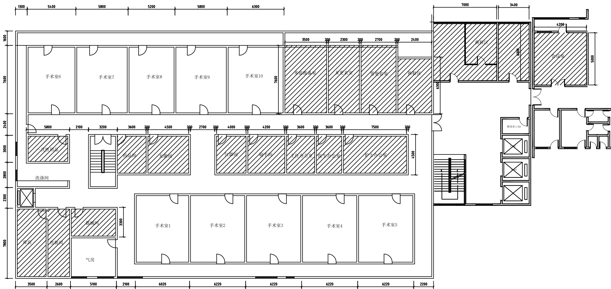
手术麻醉科东面辅助区域橡胶地板翻修平面图
